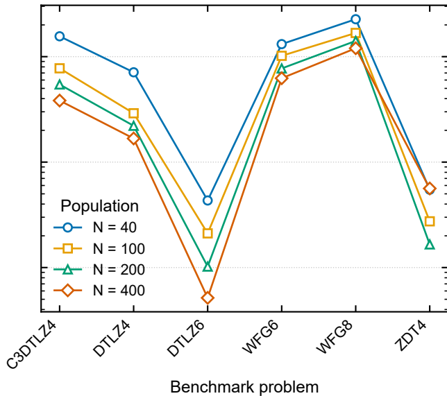
(b) PVOS-4C
